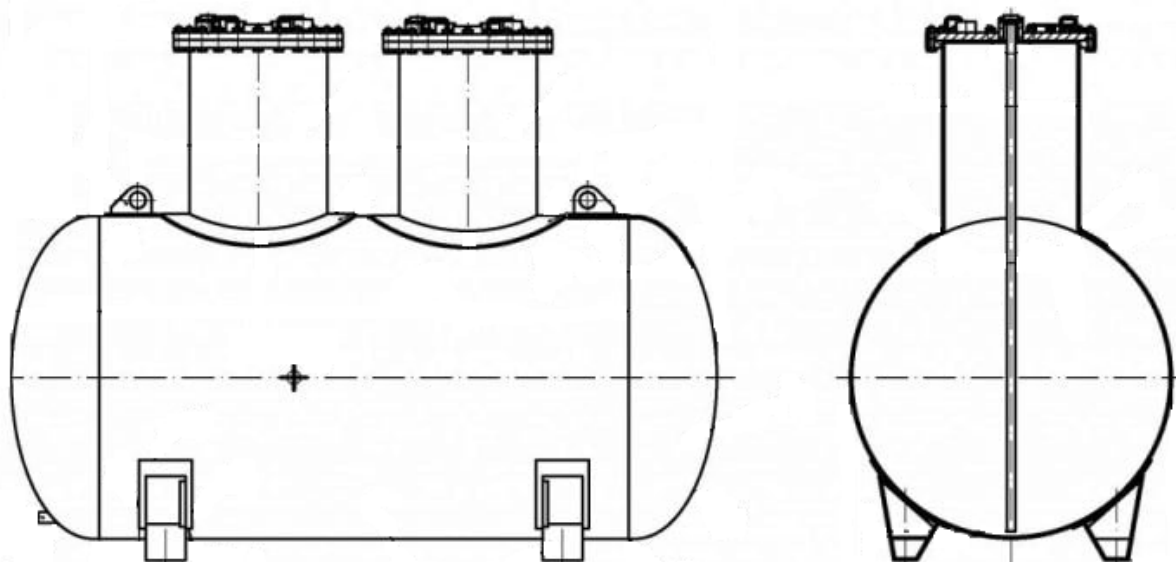
Рисунок 2 – Общий вид резервуаров РГС-25
