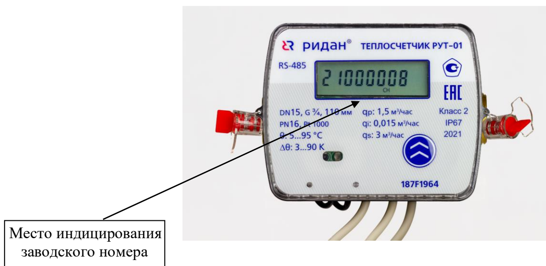
Рисунок 3 – Место индцирования заводского номера
