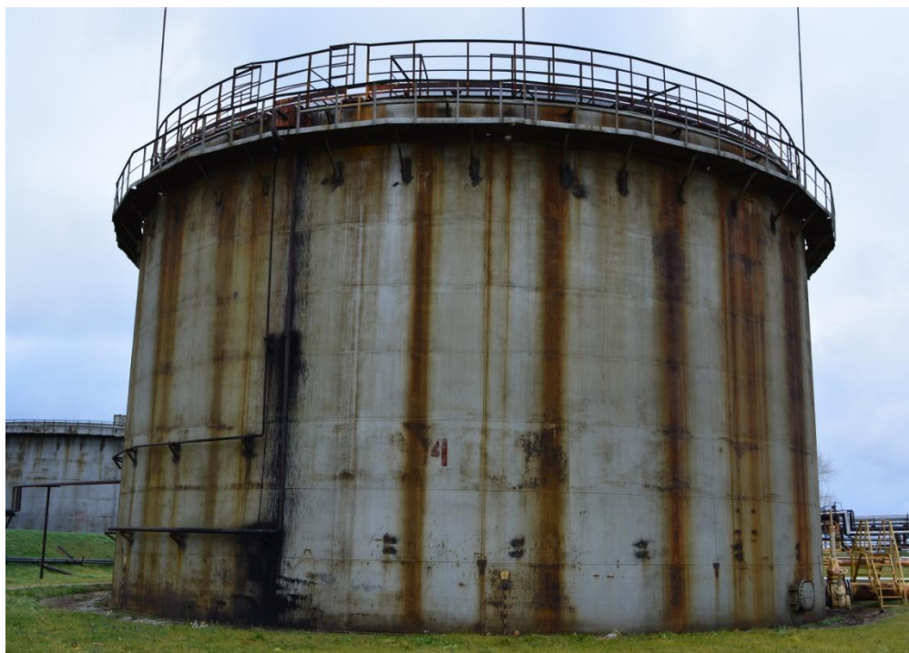
Рисунок 4 - Общий вид резервуара РВСП-5000 № 14
