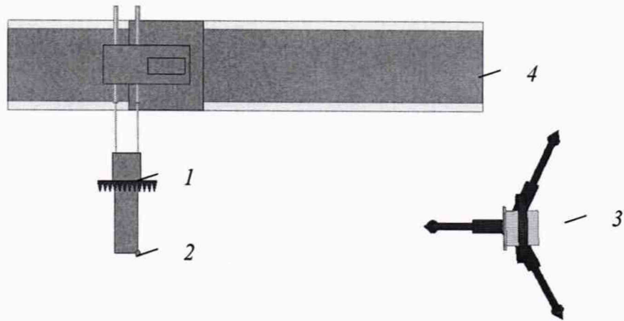
1 – антенна-зонд; 2 – оптический отражатель; 3 – система API Tracker3; 4 – сканер Рисунок 1 – Схема измерений характеристик позиционирования сканера
