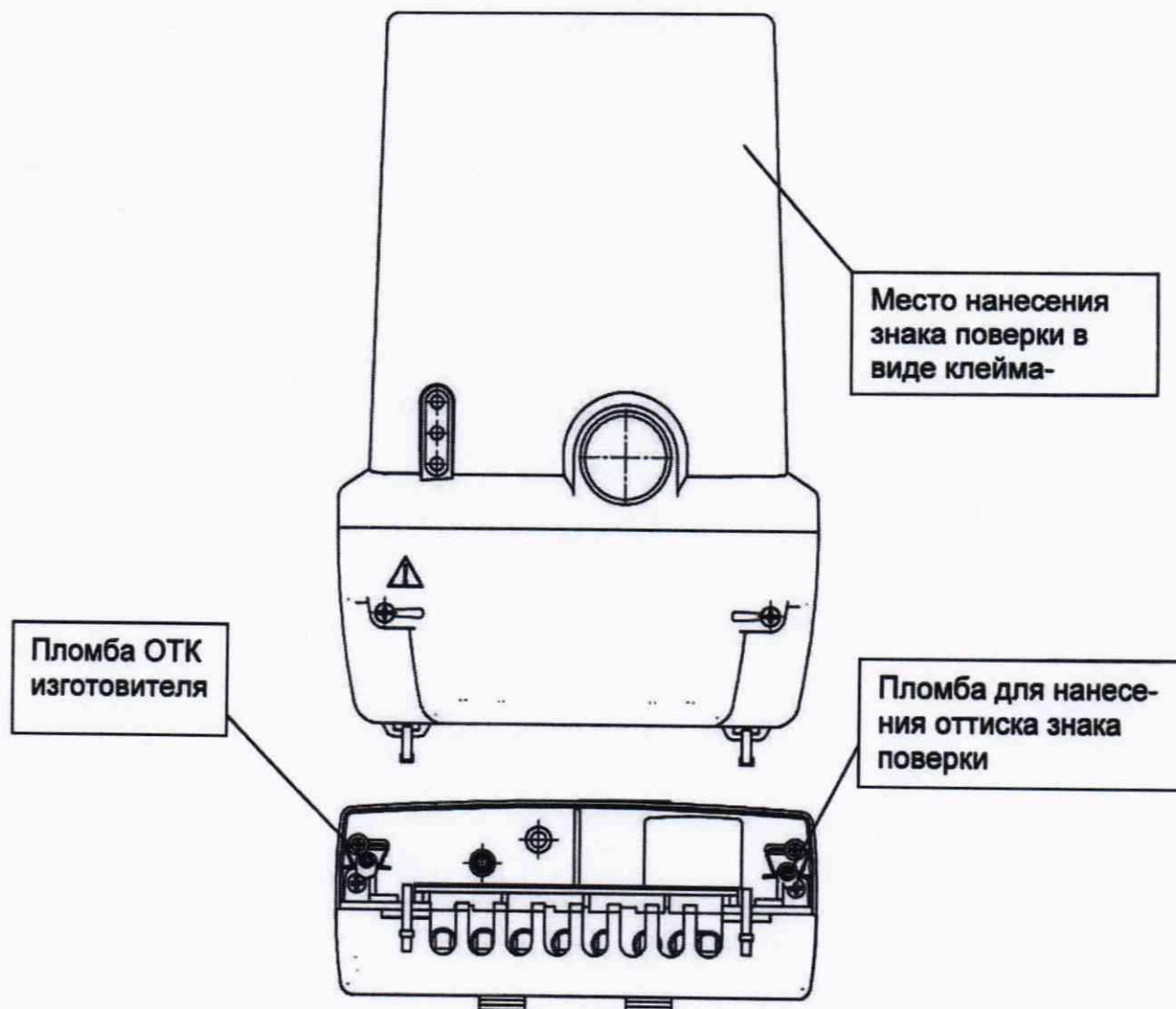
Рисунок А.5 – Корпус счетчиков СЕ318ВУ С3
