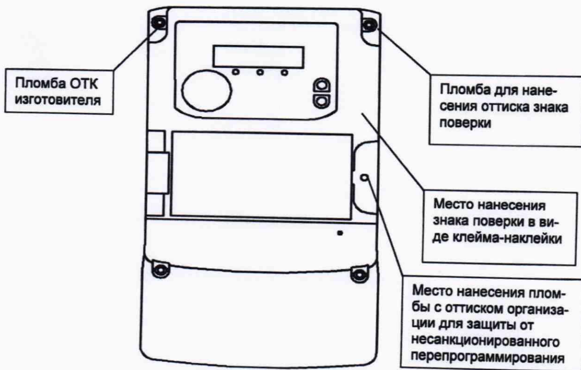
Рисунок А.3 – Корпус счетчиков CE318BY S39
