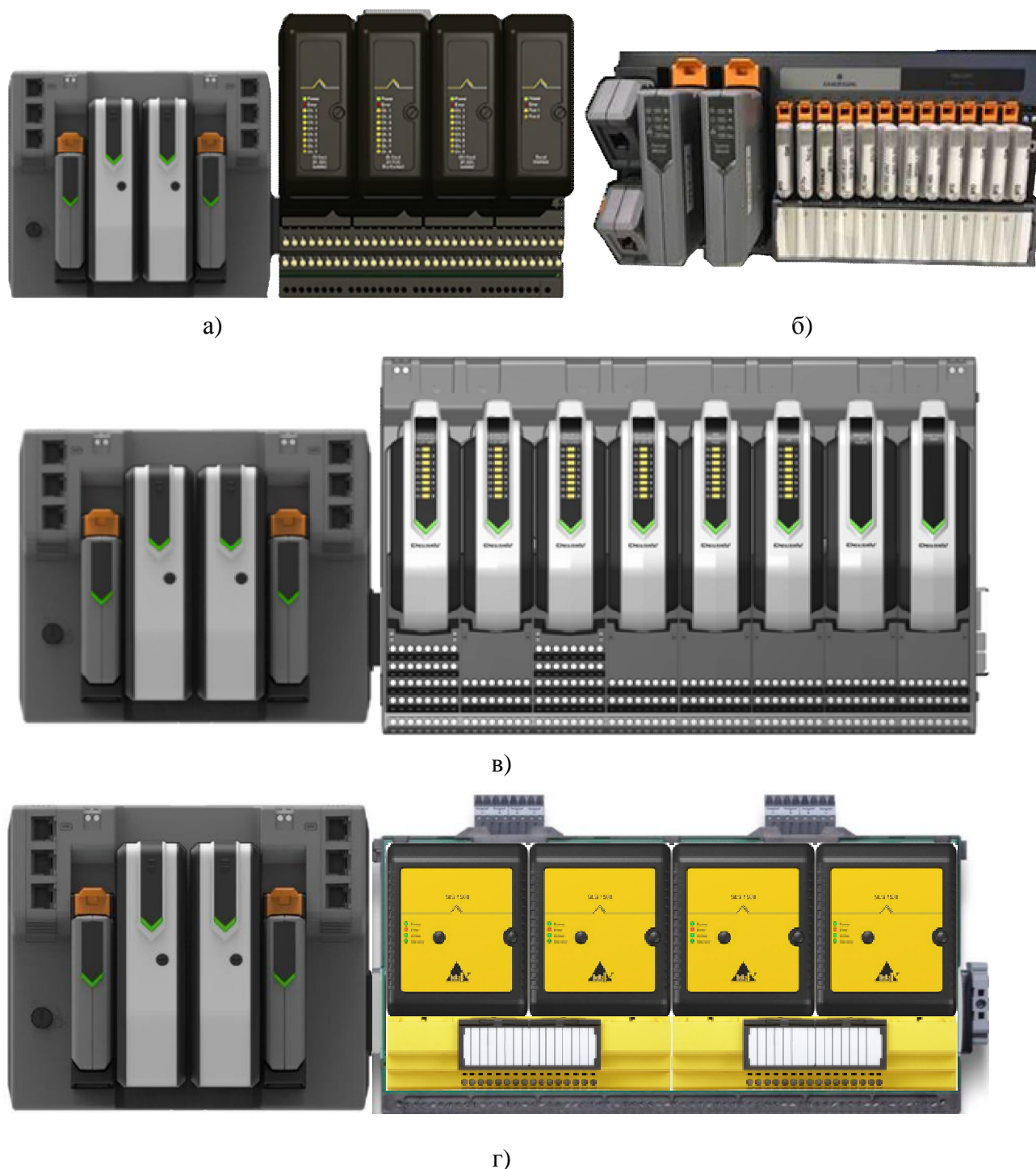
Рисунок 2 – Общий вид модулей комплексов DeltaV / ДельтаВ и DeltaV SIS / ДельтаВ ПА3: а) исполнение Р-серия для комплексов DeltaV / ДельтаВ с модулями ввода/вывода М-серии; б) исполнение S-серия, CHARM для комплексов DeltaV / ДельтаВ (горизонтального исполнения); в) исполнение Р-серия для комплексов DeltaV / ДельтаВ с модулями ввода/вывода S-серии; г) исполнение Р-серия для комплексов DeltaV SIS / ДельтаВ ПА3 с модулями ввода/вывода М-серии (модули/платы 16-канального логического вычислителя 1508).
