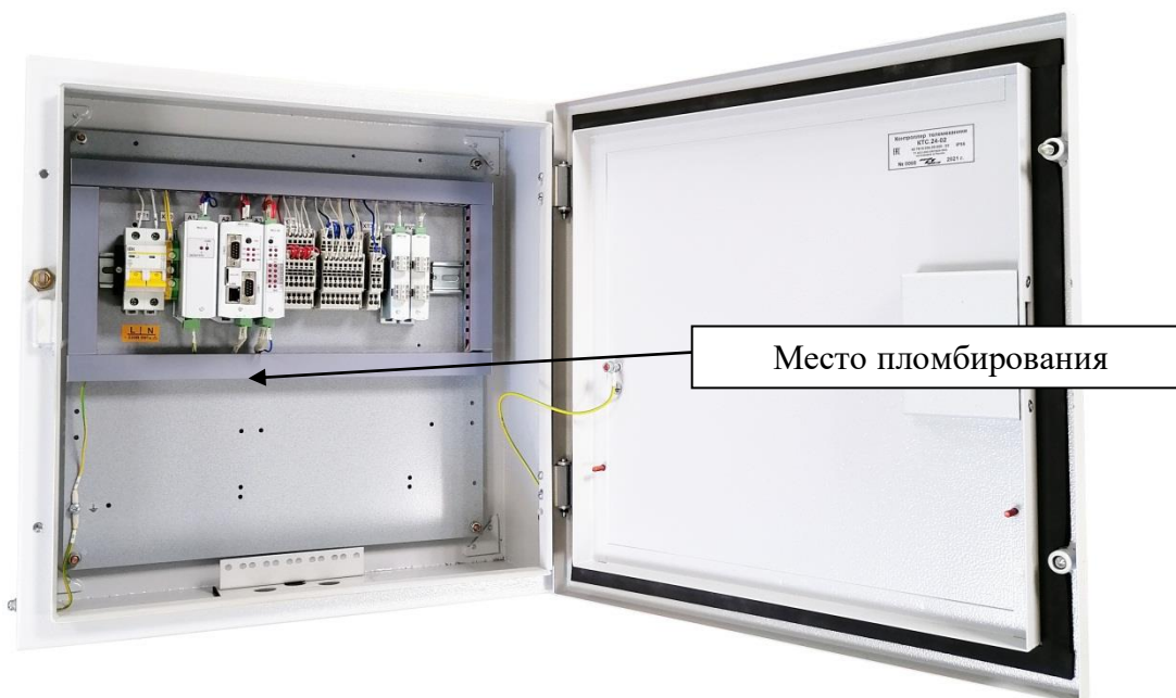
Рисунок 3 – Общий вид КТС.Х и схема пломбировки в исполнении КТС.24-02 (на базе модулей МСС 40 и МСС 08)
