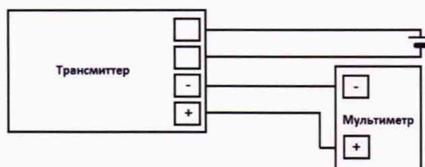
Рисунок 2 – Схема подключения приборов и средств измерения при определении отклонения действительного значения коэффициента преобразования от номинального
