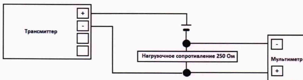
Рисунок 1 – Схема подключения приборов и средств измерения при определении относительной погрешности измерений виброперемещения
