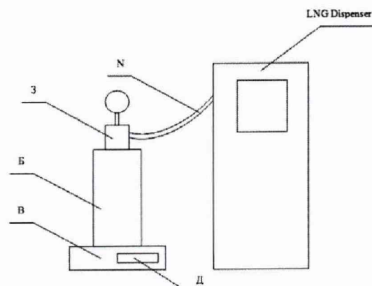
Рисунок 1 – Схема подключения колонки при проведении испытаний Обозначения: LNG Dispenser – колонка; N – раздаточный кран; Б – баллон; З – заправочное устройство с шаровым краном высокого давления и манометром; В – весы; Д – дисплей весов.
