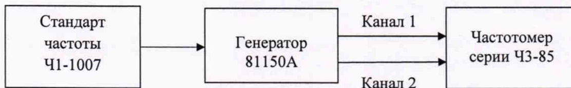
Рисунок 4 – Схема определения погрешности измерений временных интервалов
