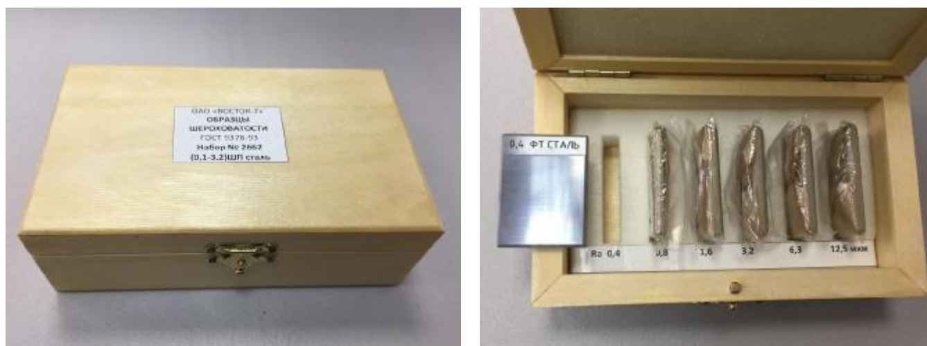
Рисунок 1 - Общий вид наборов образцов шероховатости поверхности (сравнения) модификации В7-1833
