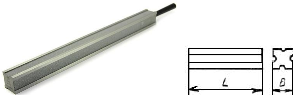
Рисунок 3 – Общий вид, обозначение основных размеров линеек ЛЧ
