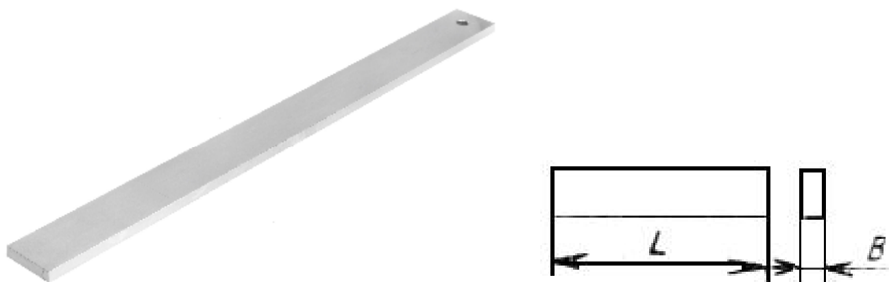
Рисунок 4 – Общий вид, обозначение основных размеров линеек ШП
