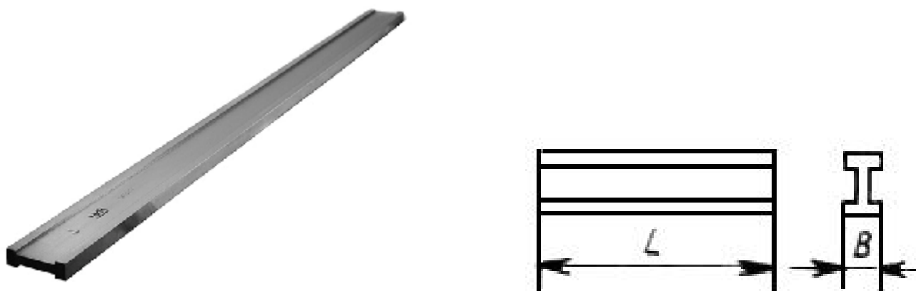
Рисунок 5 – Общий вид, обозначение основных размеров линеек ШД
