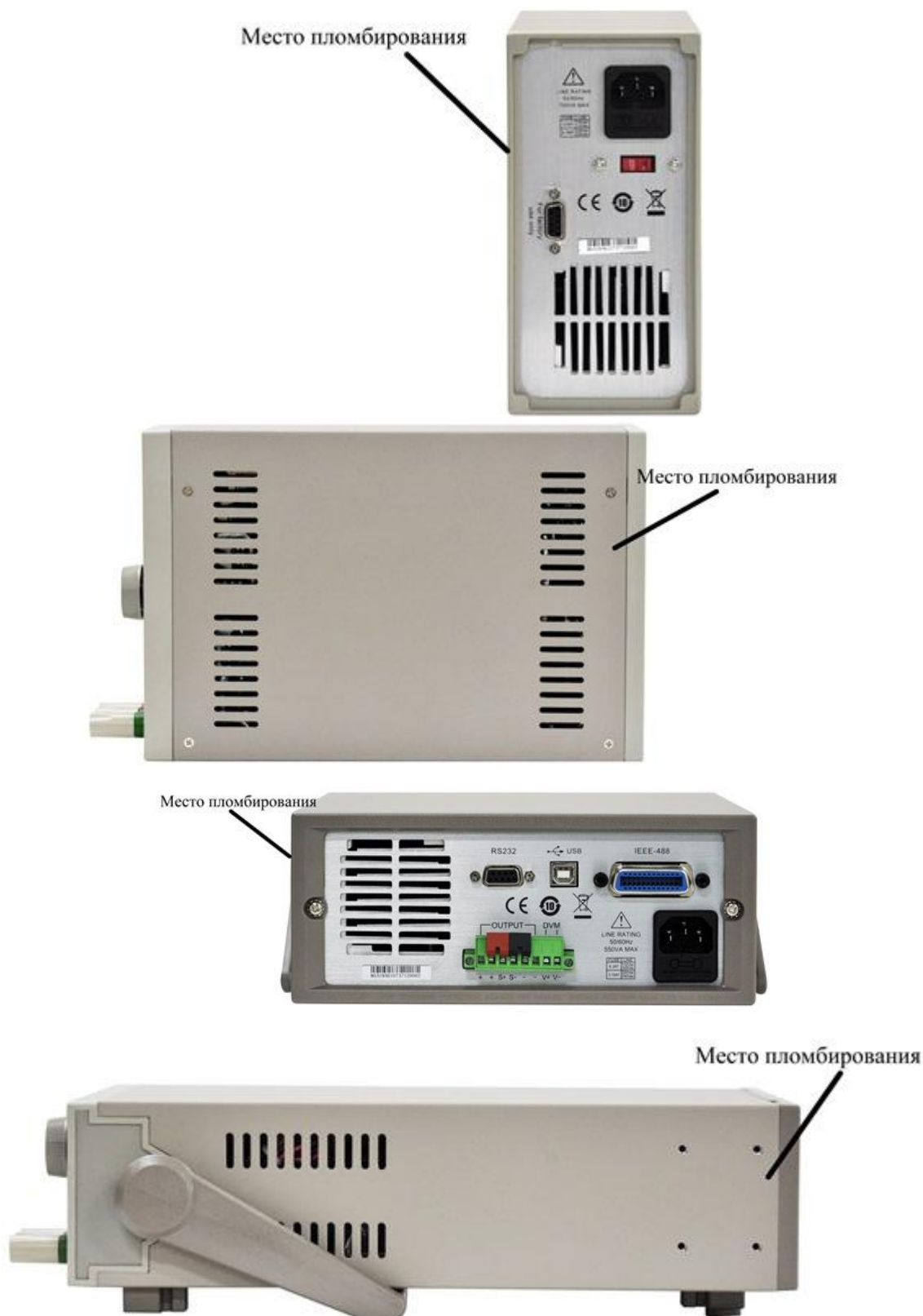
Рисунок 2 – Схема пломбирования источников от несанкционированного доступа
