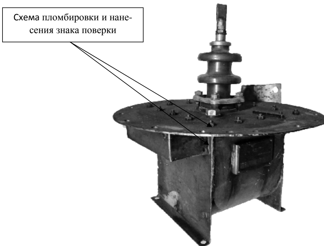
Рисунок 1 – Общий вид трансформаторов напряжения и схема пломбировки от несанкционированного доступа
