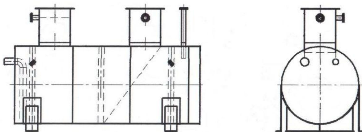
Рисунок 1 – Эскиз общего вида резервуара ЕП-8-2000-1300-3
