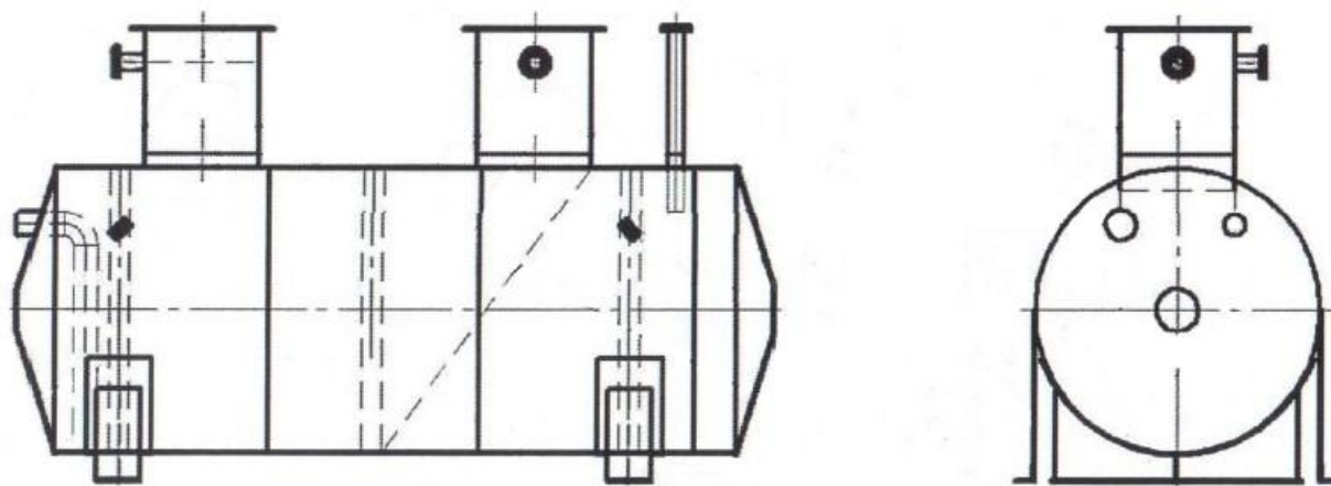
Рисунок 1 – Эскиз общего вида резервуаров ЕП-16
