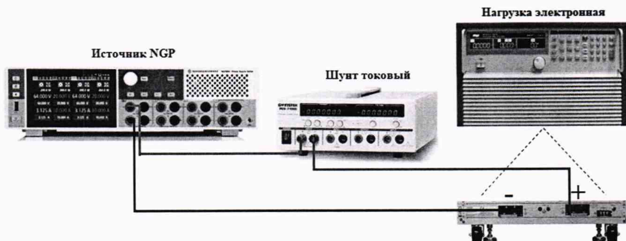
Рисунок 5 – Структурная схема соединения приборов для определения нестабильности силы тока на выходе источников
