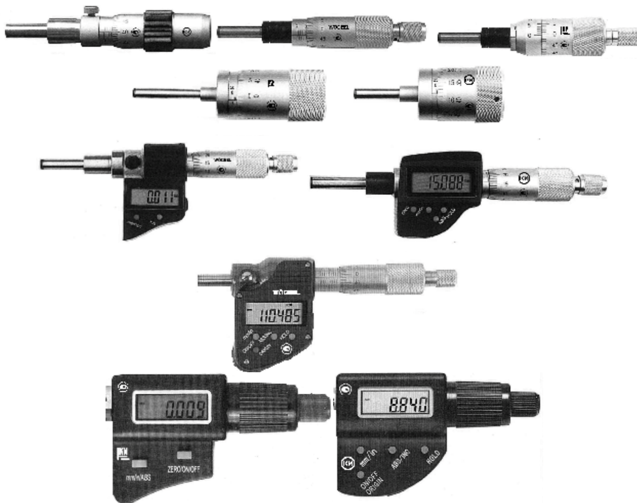
Рисунок 6 – Общий вид микрометров МГ, МГ Ц
