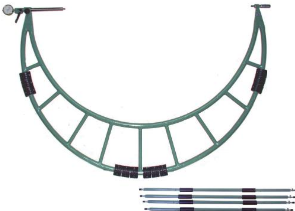
Рисунок 3 - Общий вид микрометров рычажных МРИ 1200 - МРИ 2000
