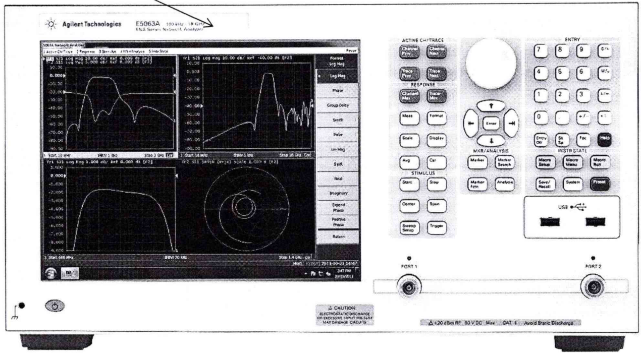
Рисунок 1 – Общий вид анализатора E5063A. Вид спереди
