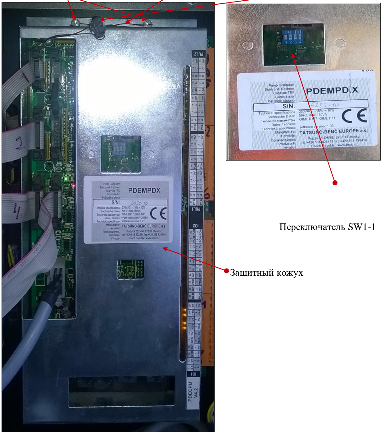
Рисунок 3 – Пломбировка суммарного электронного счетчика и положение фискального переключателя (SW1-1)
