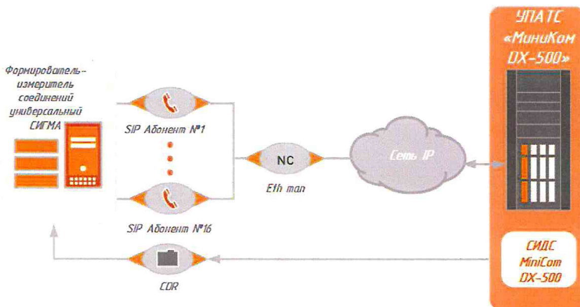
Рисунок 1- Схема поверки
