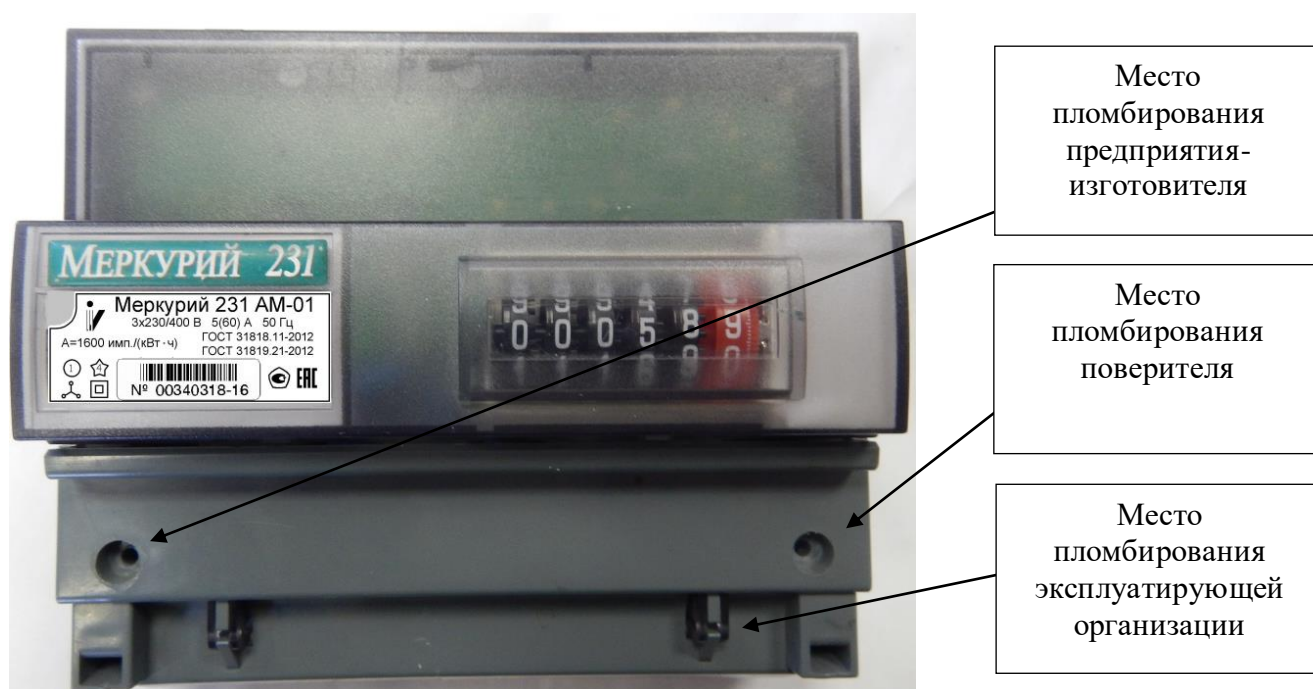
Рисунок 1 – Общий вид счетчиков «Меркурий 231 AM-0X», «Mercury 231 AM-0X» с указанием мест пломбирования и нанесения знака поверки
