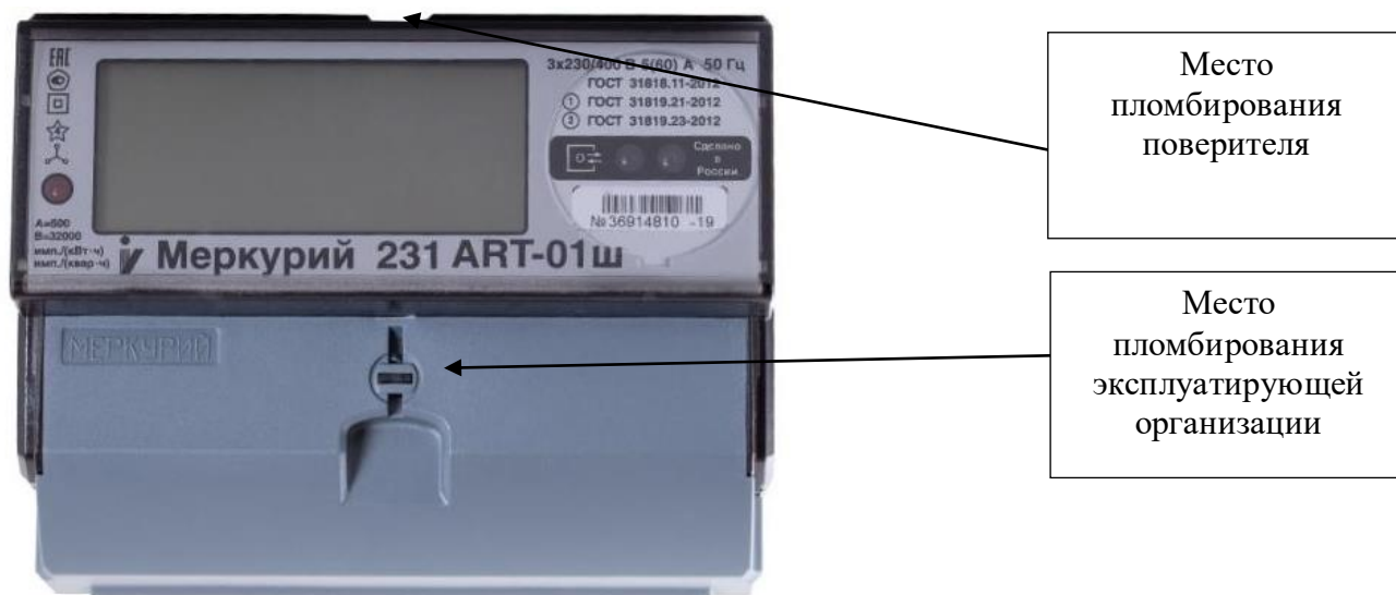
Рисунок 4 – Общий вид счетчиков «Mercury 231 ART-0Xш», «Mercury 231 ART-0Xш» с указанием мест пломбирования и нанесения знака поверки
