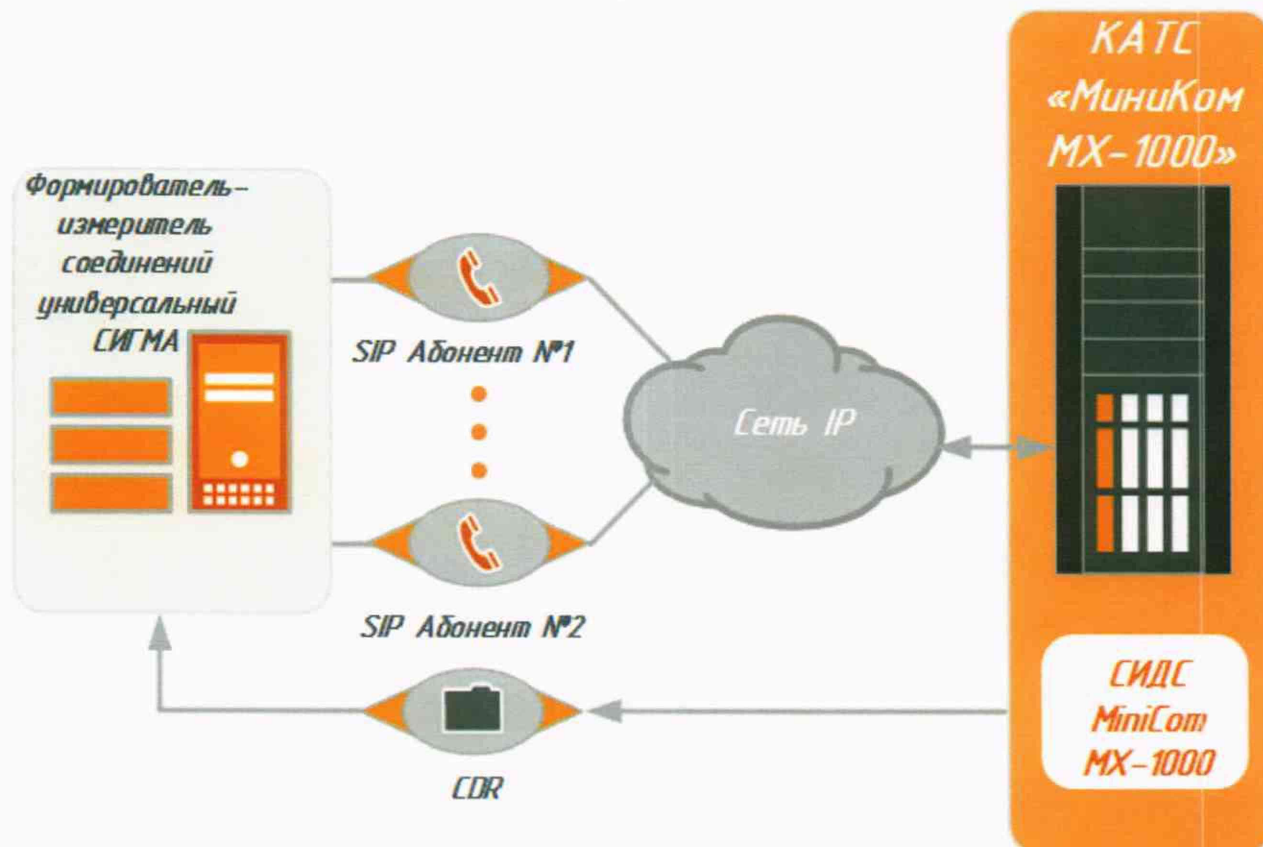
Рисунок 1- Схема поверки
