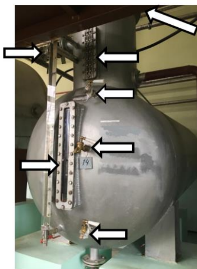
Рисунок 2 – Схема пломбировки мерника М1кл, зав.№ 2851297 от несанкционированного доступа, обозначение места нанесения знака поверки
