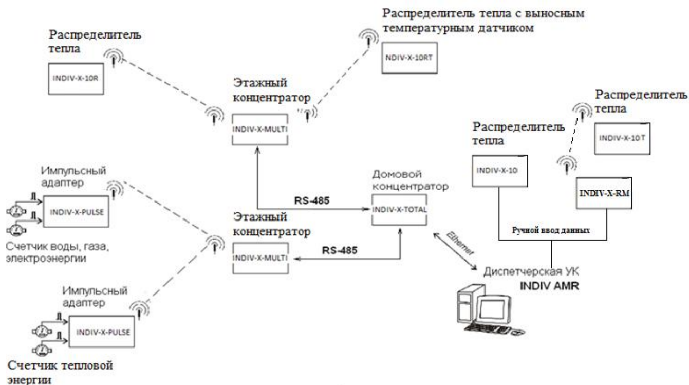
Рис.1 – Структурная схема системы автоматизированной измерительной количества энергоресурсов INDIV-X-AMR
