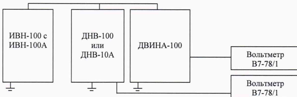
Рисунок 1 - Проверка погрешности измерений напряжения постоянного тока
