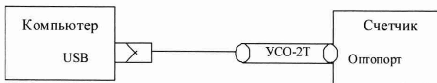
Рисунок Б.2- Схема подключения счётчика к компьютеру через оптопорт
