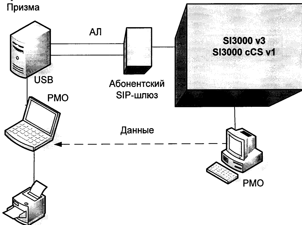
Рисунок 3. Схема испытаний СИДС
