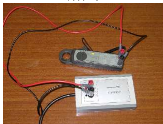
Рисунок 7 - Комплект измерения тока с токовыми клещами ТК-200DC «/200DC»
