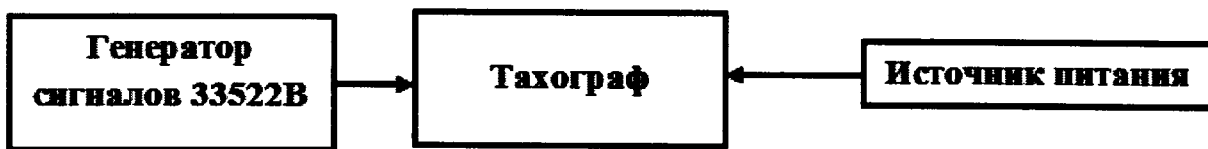
Рисунок 4 – Схема проведения измерений при определении инструментальной погрешности измерения скорости по датчику движения
