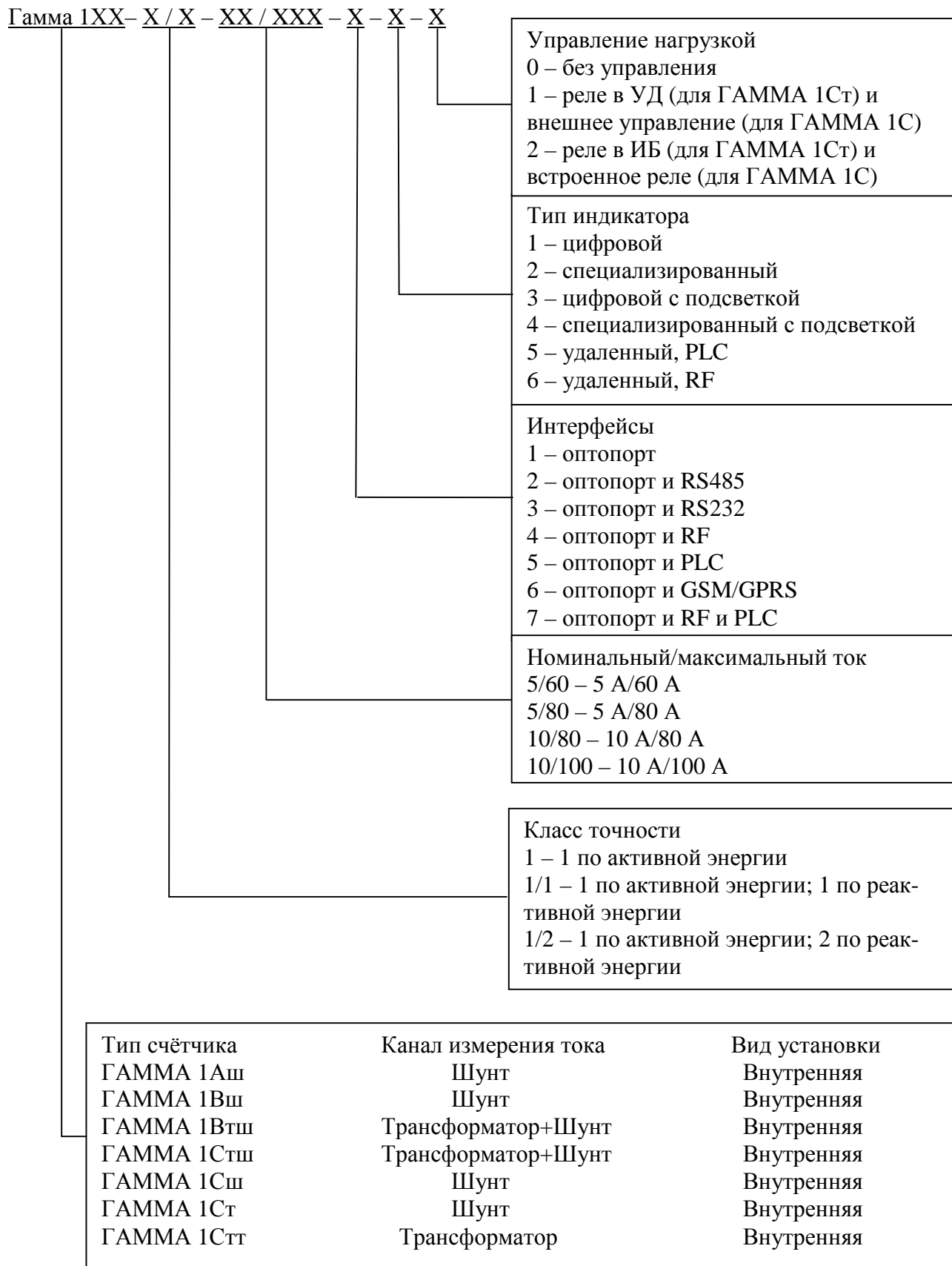
Рисунок 1 - Структура условного обозначения счётчиков
