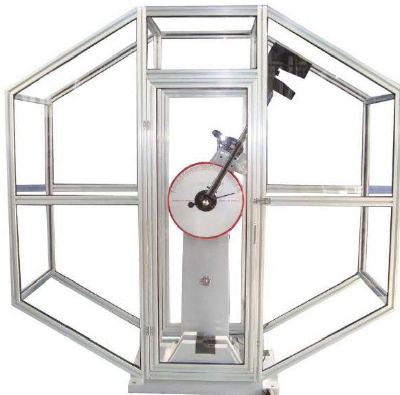
Рисунок 2 - Общий вид копров маятниковых КМ-300, КМ-450, КМ-500
