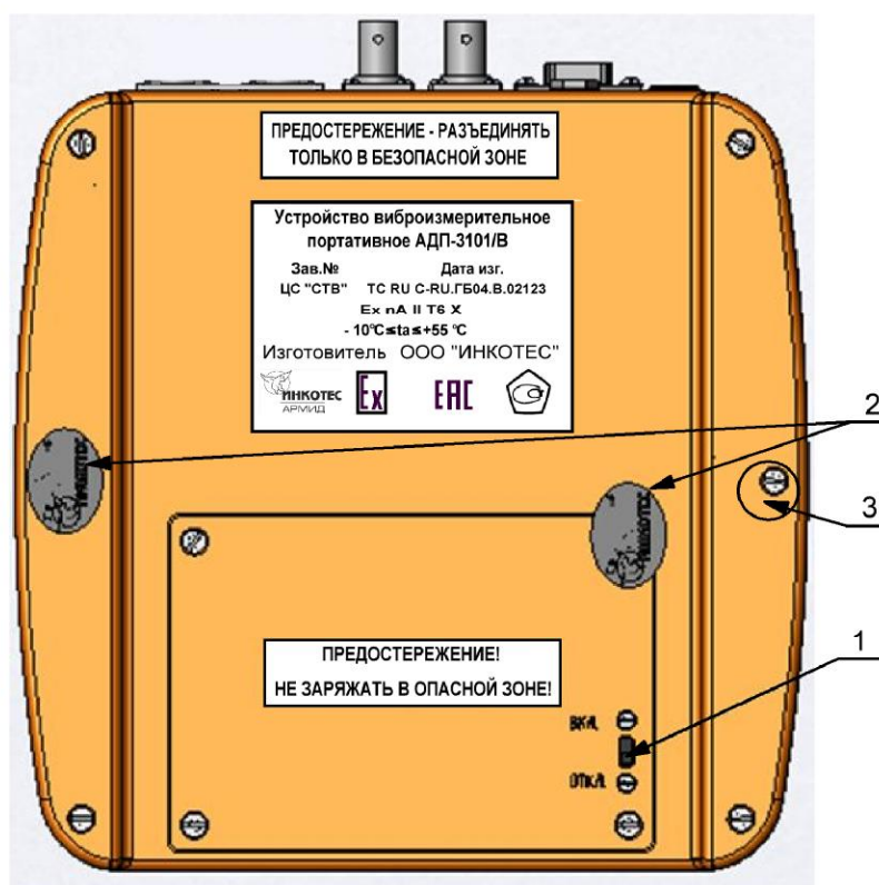
Рисунок 2 - Вид блока измерения и индикации прибора АДП-3101 с пломбировочными стикерами и указанием мест нанесения знака поверки: 1- тумблер отключения аккумуляторного блока; 2-места установки пломб изготовителя; 3-место нанесения знака поверки.
