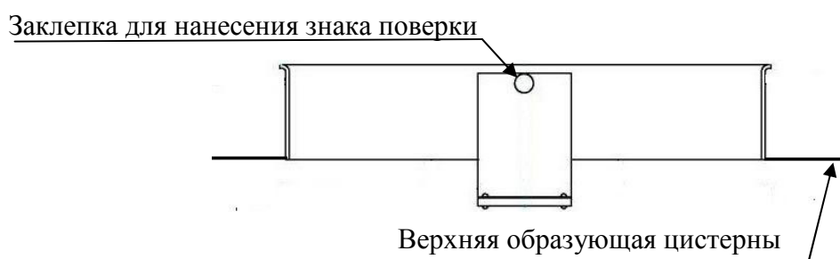
Рисунок 5 – Схема пломбировки от несанкционированного изменения положения указателя уровня налива в полости цистерны модификации БК, обозначение места нанесения знака поверки
