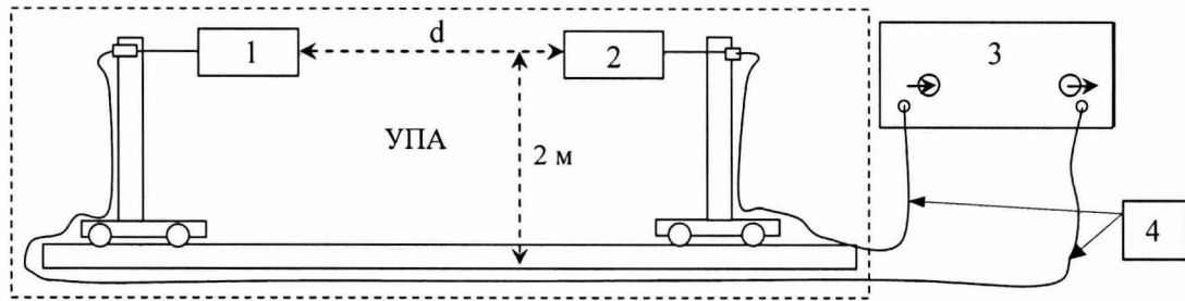
УПА – установка перемещения антенн; 1 – излучатель; 2 – измерительная антенна; 3 – измерительный приемник ESPIЗ с трекинг-генератором из состава РЭИА-1; 4 – соединительные кабели из состава РЭИА-1.
