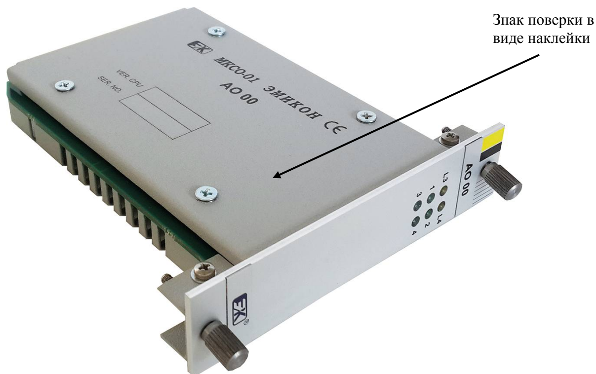
Рисунок 2 - Общий вид модулей ввода-вывода с обозначением места нанесения знака поверки
