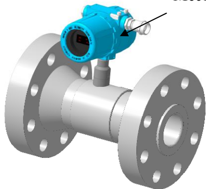
Рисунок 1 - Исполнение фланцевое, уплотнение прокладками или кольцами
