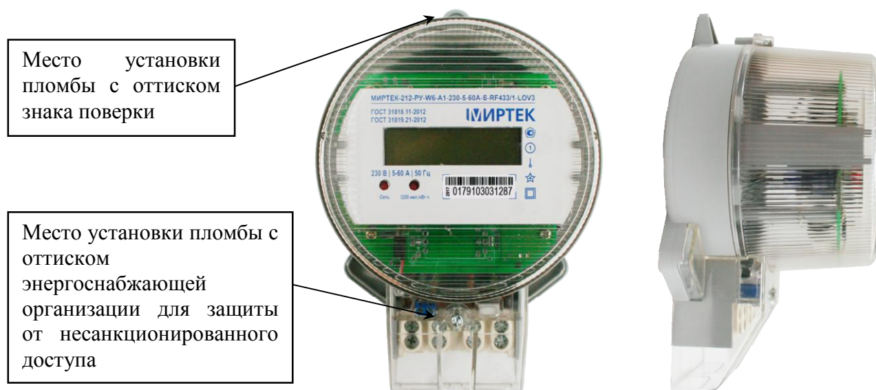
Рисунок 4 - Общий вид счетчика и схема пломбировки от несанкционированного доступа в корпусе типа W6
