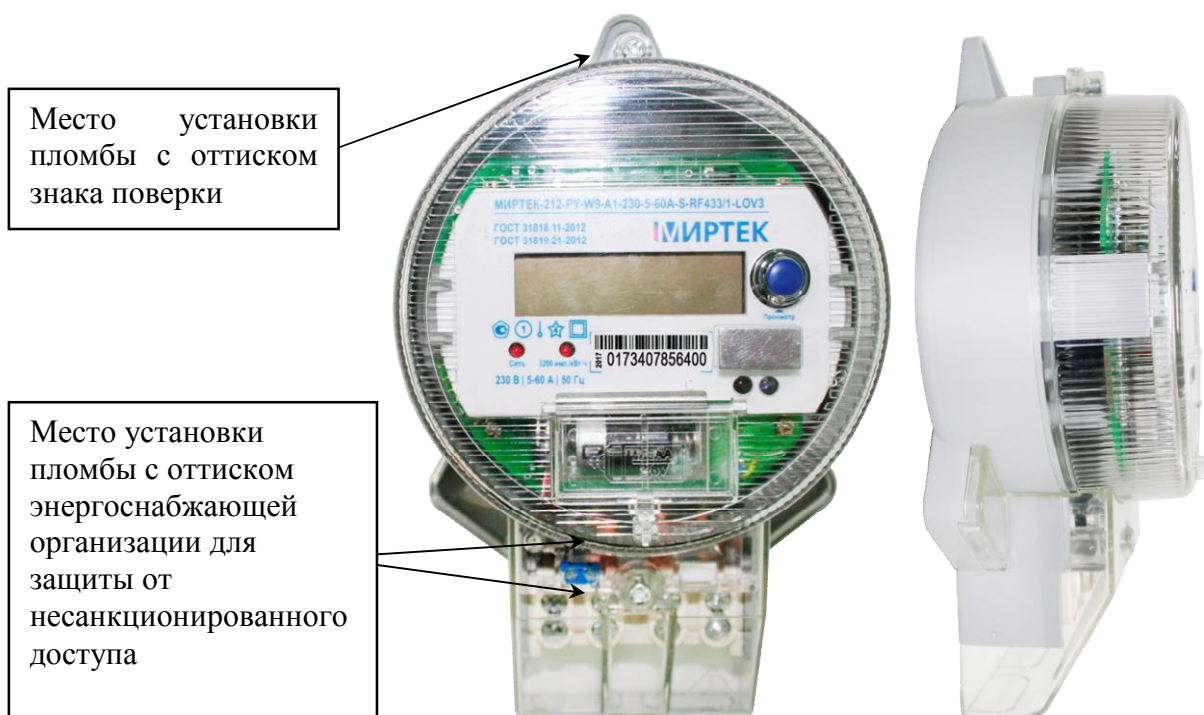
Рисунок 6 - Общий вид счетчика и схема пломбировки от несанкционированного доступа в корпусе типа W9
