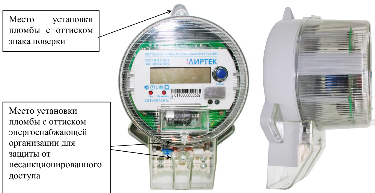
Рисунок 5 - Общий вид счетчика и схема пломбировки от несанкционированного доступа в корпусе типа W6b
