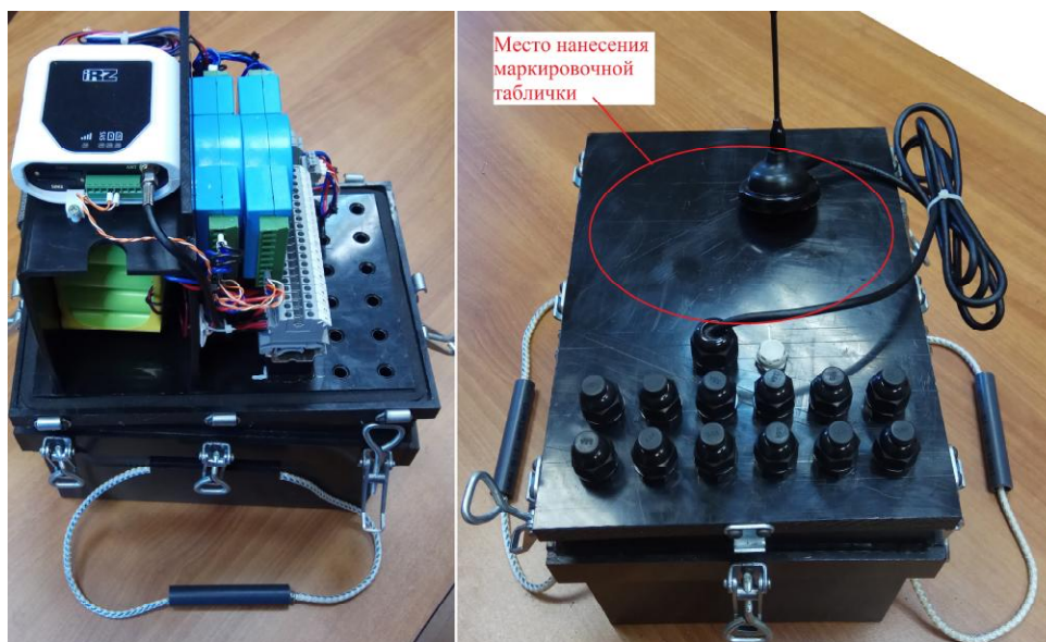
Рисунок 2 – Общий вид корпуса блока управления АИП на примере модификации IV-F
