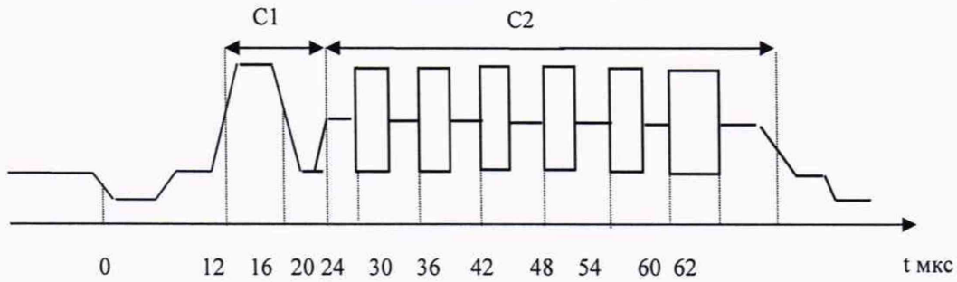
Рисунок А.2 - Сигнал II по ГОСТ 18471
