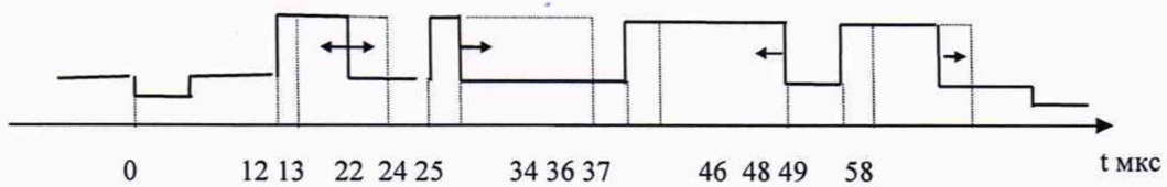
Рисунок А.5 - Сигнал Y по ГОСТ 18471
