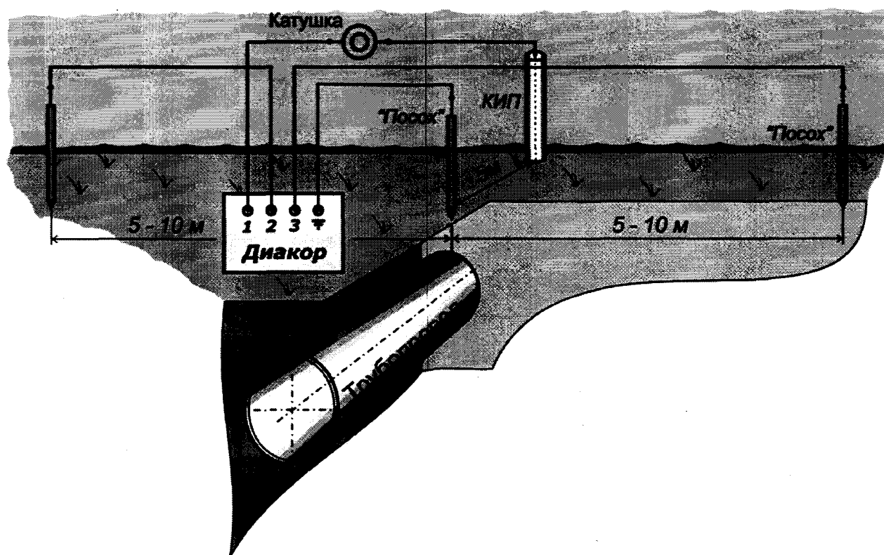
Рисунок 3.1.2.3.2.1 – Трехэлектродный метод
