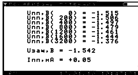
Рисунок 2.8.3.4 – Окно «ИПП - расчетные значения I_{pp} »
