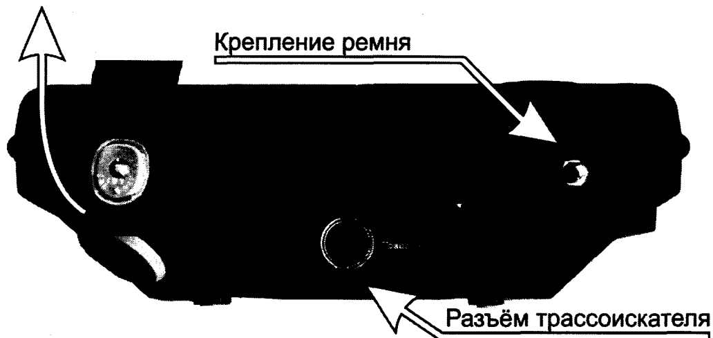
Рисунок 2.1.3 – Вид справа
