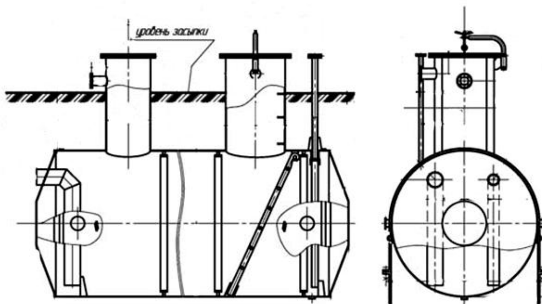
Рисунок 2 - Эскиз резервуара
