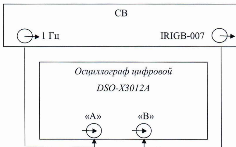
Рисунок 4 – Схема для определения задержки выдачи телеграммы IRIGB-007 через порт RS-422 относительно формируемой ШВ
