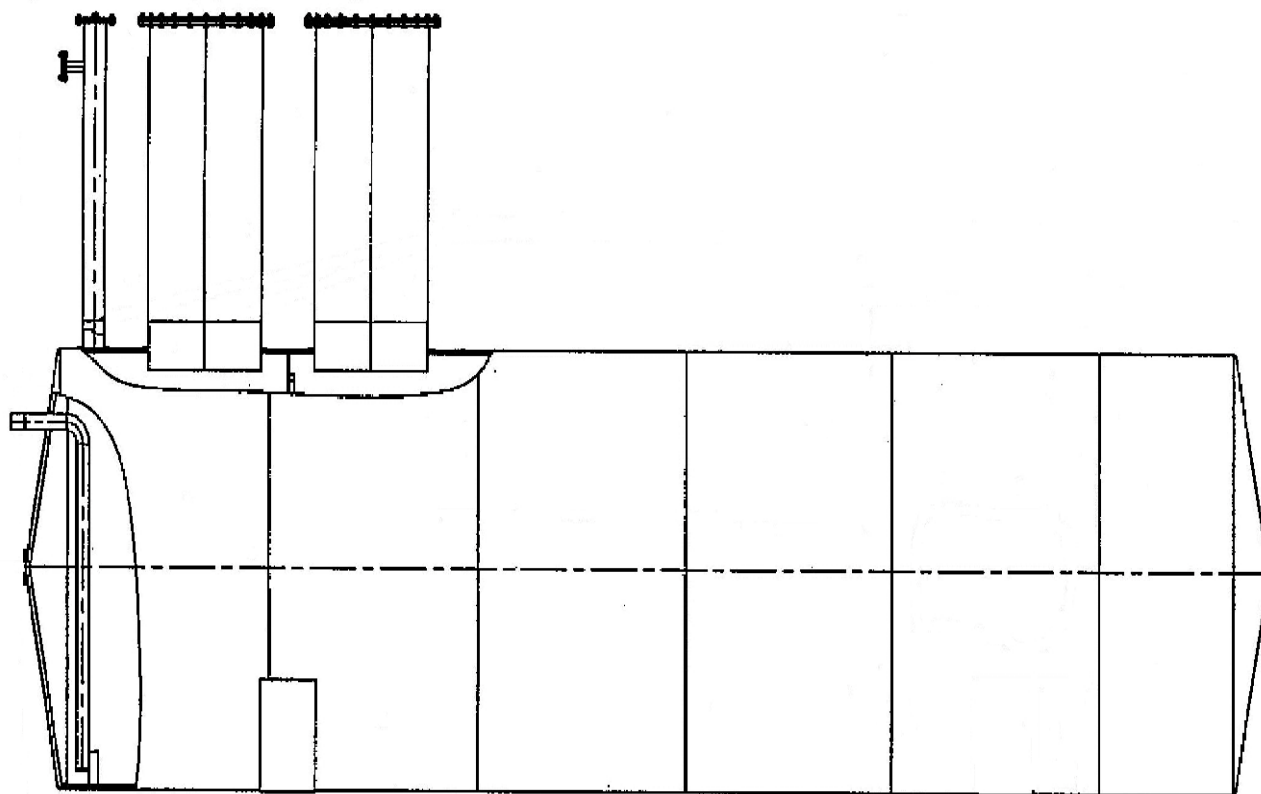
Рисунок 1 - Общий вид резервуаров стальных горизонтальных цилиндрических РГС-40
