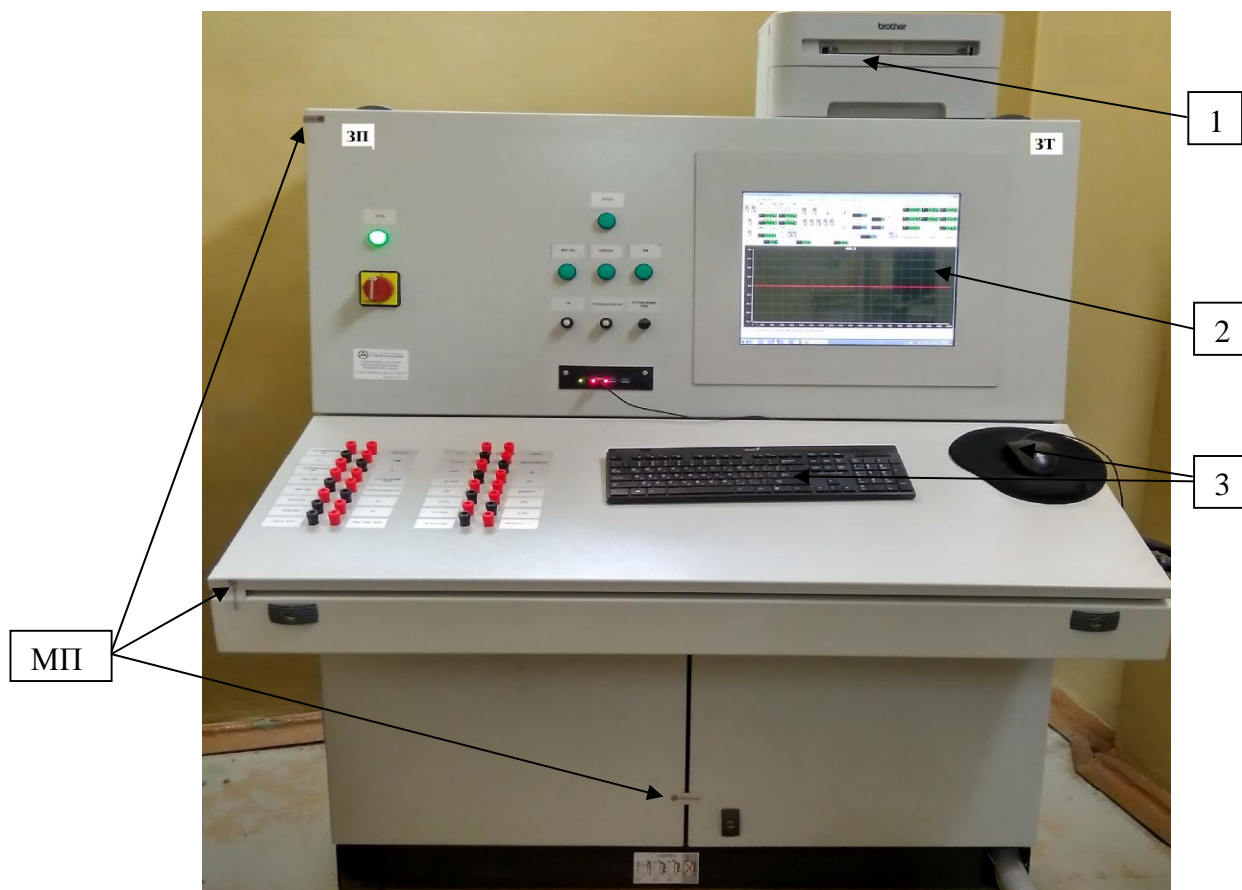
1 – лазерное печатающее устройство Brother HL-2132; 2 – сенсорный резистивный монитор EASY MOUNT 17 TG1701W4EM; 3 – клавиатура с манипулятором типа «мышь» Genius Slim Star 18150
