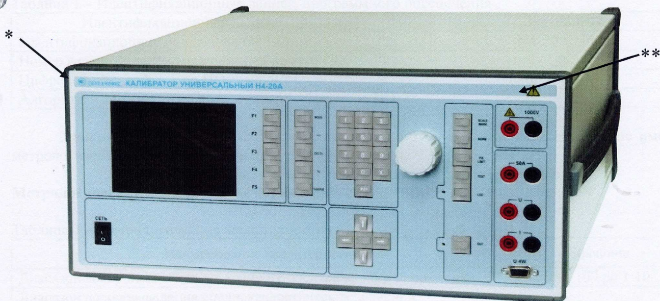
Рисунок 1 – Калибратор универсальный Н4-20А
