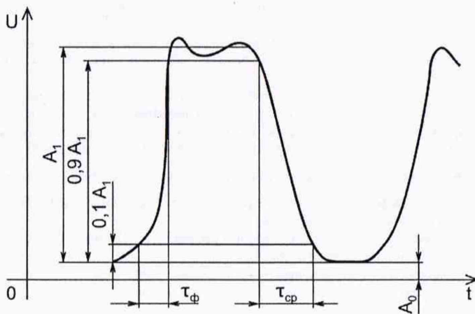
Рисунок 6.6 – Сигнал прямоугольной формы
