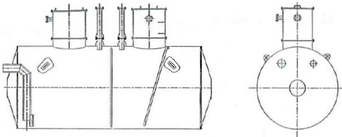
Рисунок 1 - Общий вид эскиза резервуара РГС-25
