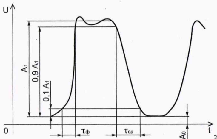
Рисунок 6 – Сигнал прямоугольной (ТТЛ) формы
